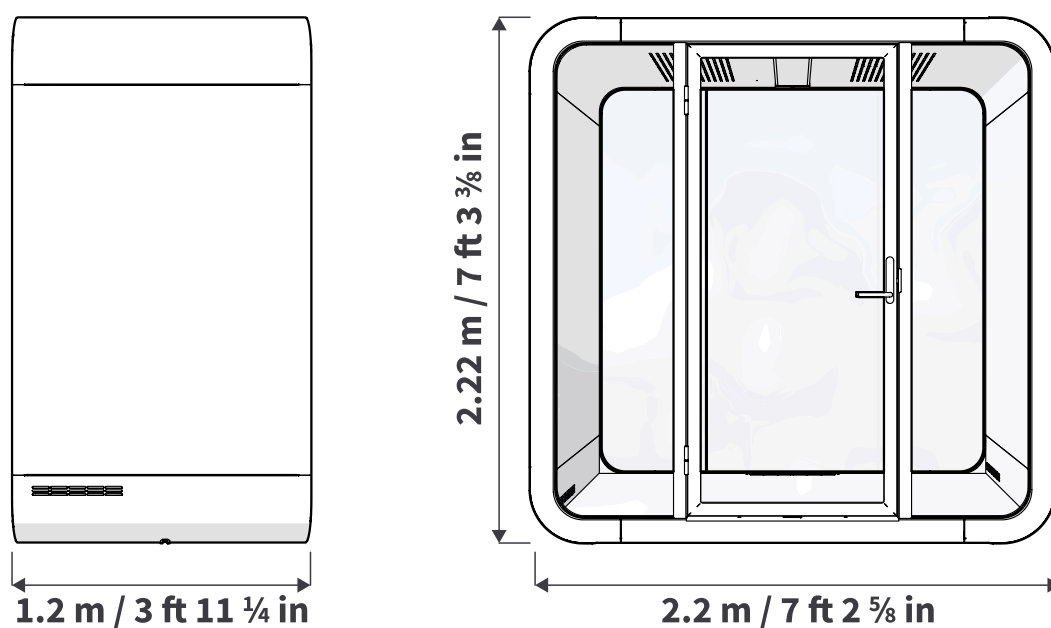
Illustration 2 : Dimensions principales de la cabine
