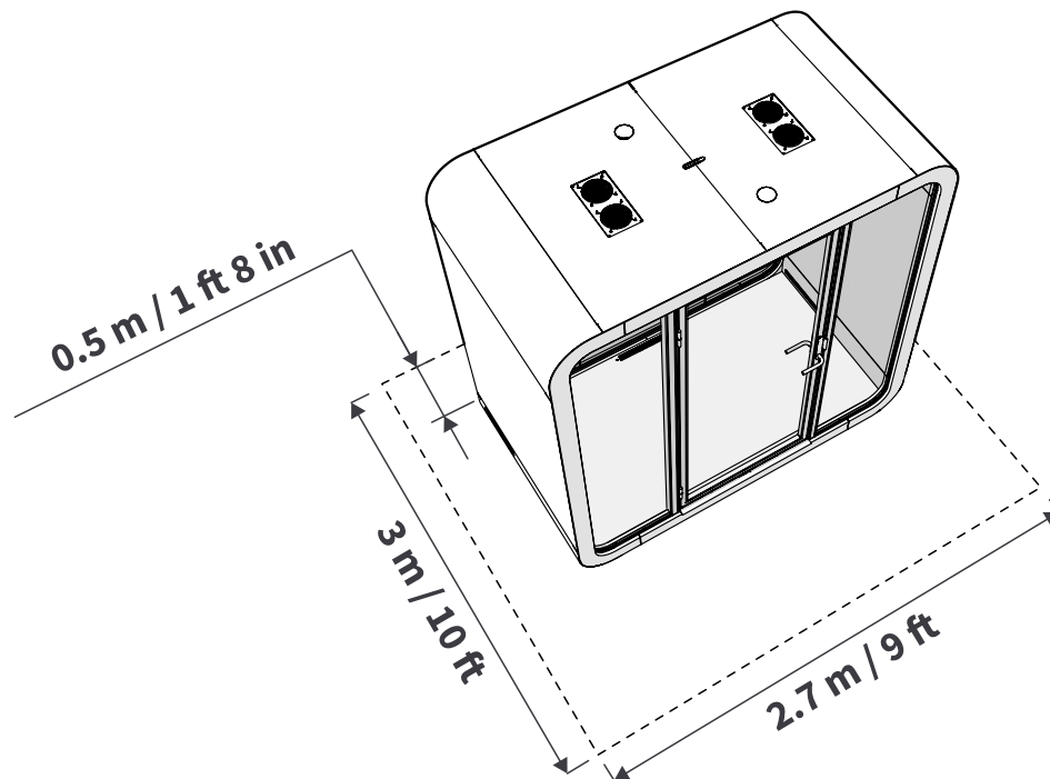
Illustration 3 : Dimensions de l'espace d'installation
