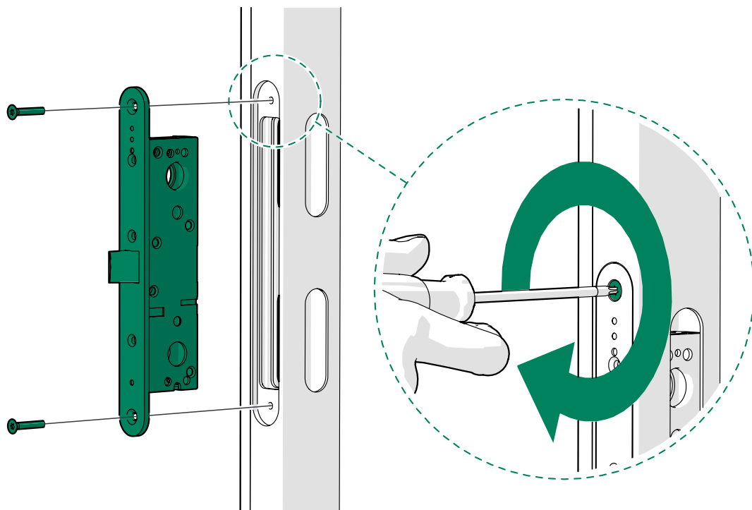
Illustration 5 : Boîtier de serrure standard
