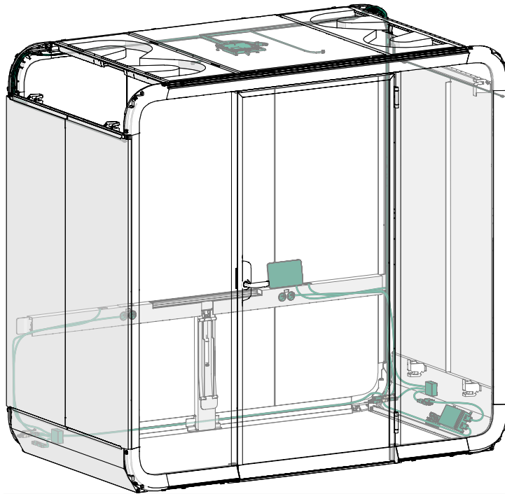
Figura 4: Vista general del sistema eléctrico de la cabina
