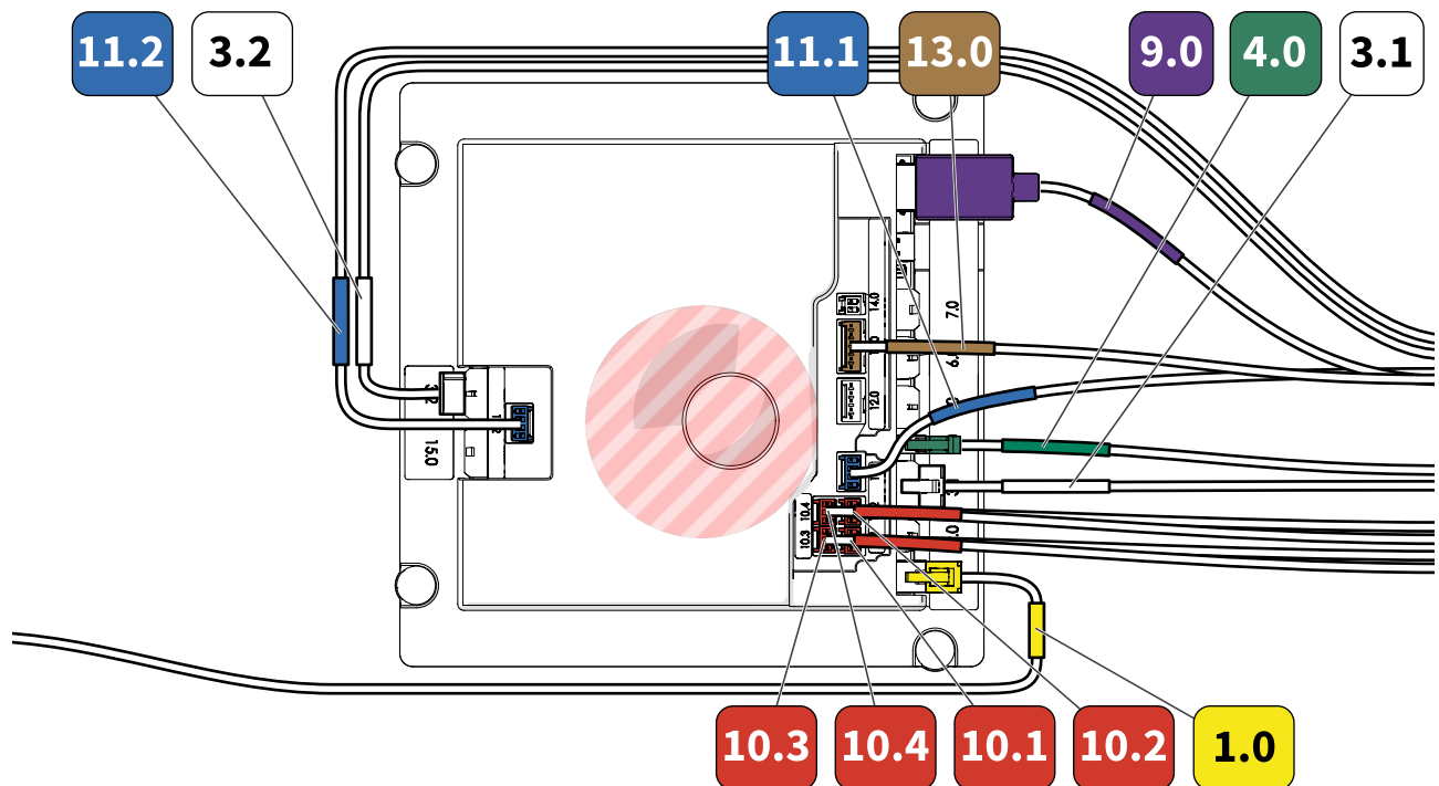
Figura 6: Etiquetas de los conectores de la unidad central
