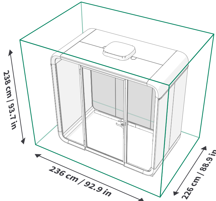
Figura 2: Espacio operativo necesario
